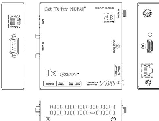
HDC-TH100-D
